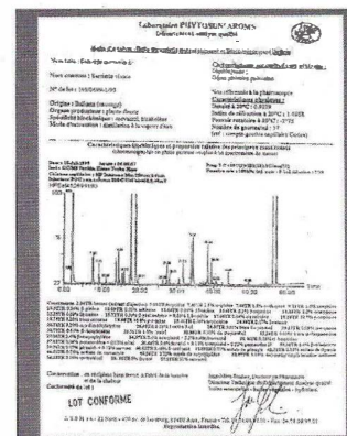
Figura 1. Perfil cromatográfico de una muestra de aceite esencial de Satureia montana
